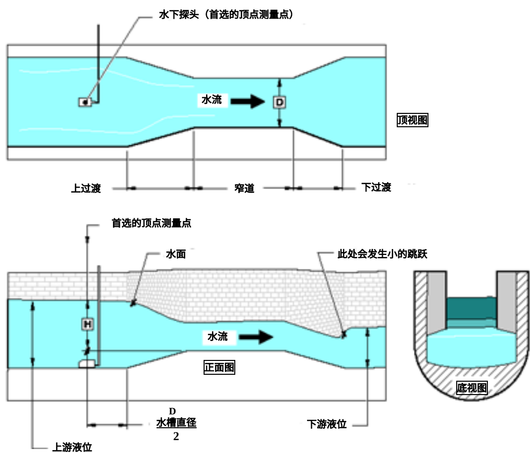
图 53 Leopold-Lagco 型水槽
