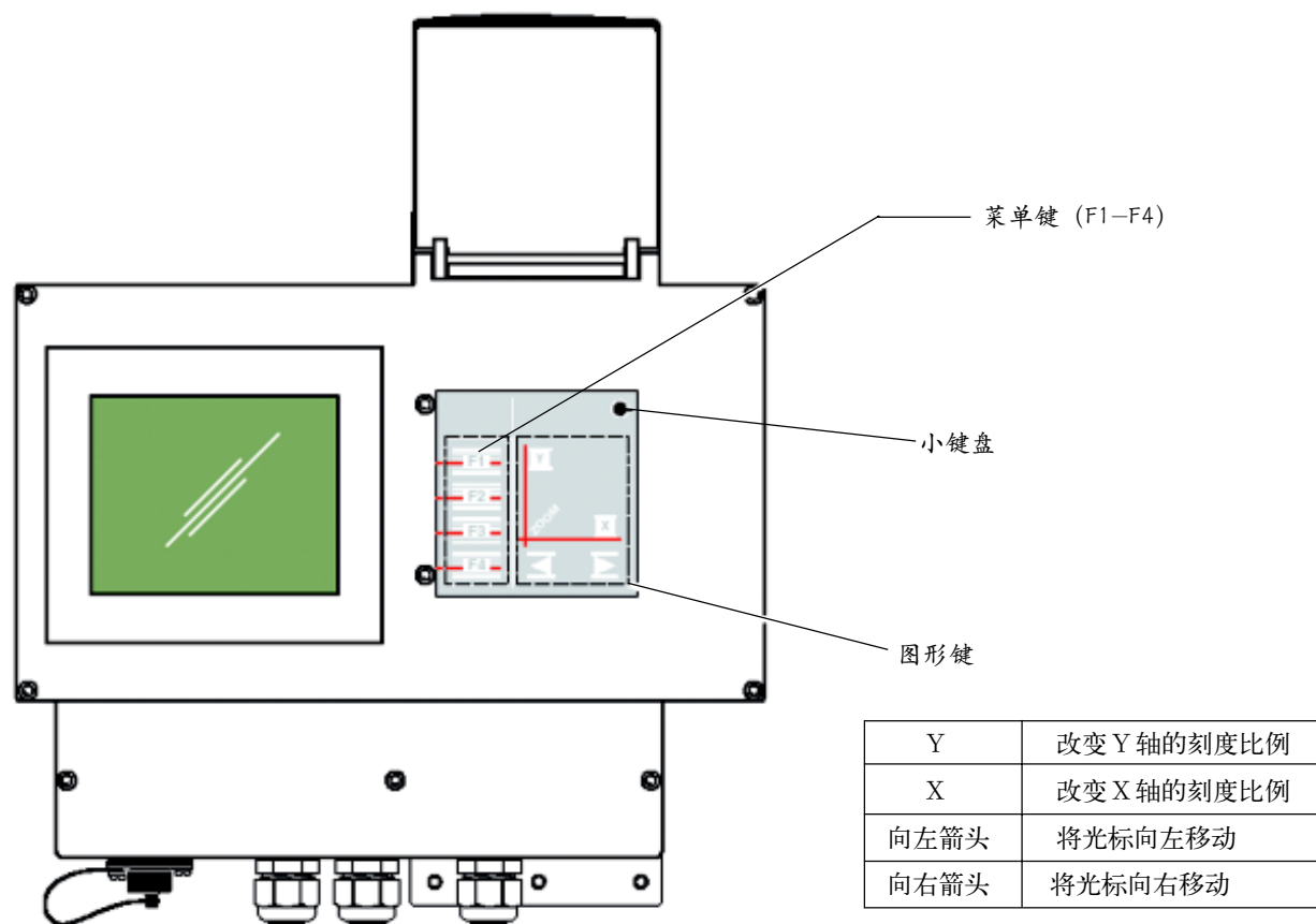
图 3 在 OptiQuant 污泥界面监视仪上各个键的位置
