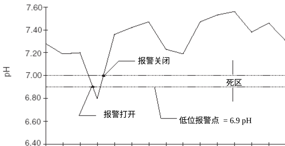
图 31 死区的概念
